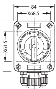
3-контактный
